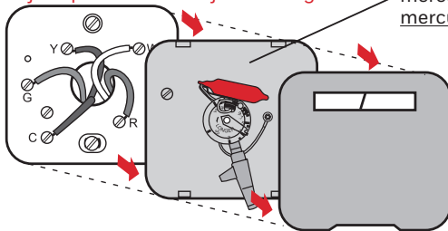
Termostato viejo
