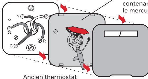
Ancien thermostat
